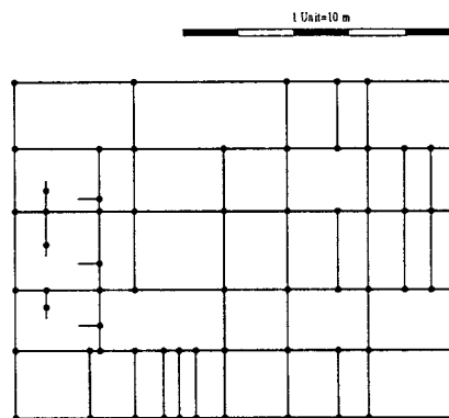
Fig. 1.—E.R. Balaídos II: Vista en planta de la malla de tierra. (Se indica con puntos negros la situación de las picas).
