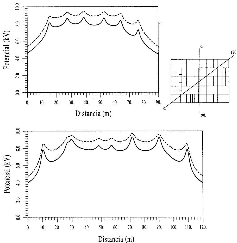
Fig. 2.—E.R. Balaídos II : Perfiles de Potencial en la superficie del terreno a lo largo de las diferentes líneas indicadas. (En trazo continuo se representan los resultados obtenidos con el modelo de terreno de dos capas, y con trazo discontinuo los del modelo uniforme).
