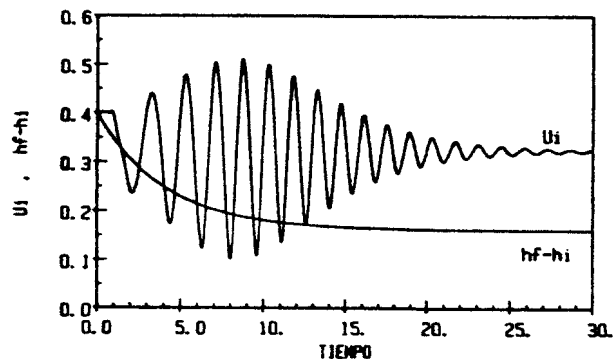
Figura 4: evolución temporal de la velocidad u_i , debida a un decaimiento exponencial del subenfriamiento de entrada.
