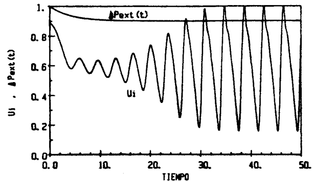
Figura 6: evolución temporal de la velocidad u_i , debida a un decaimiento exponencial del salto externo de presión.
