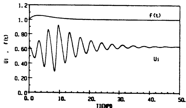
Figura 5: evolución temporal de la velocidad u_i , debida a una oscilación en el flujo de calor.
