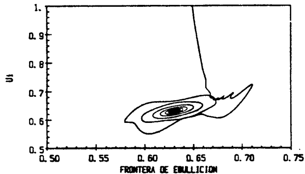
Figura 2: proyección de la trayectoria en el plano \lambda - u para un comportamiento estable ( Ne_{ub}=7.57, Np_{cb}=12, Fr=0.0837, K_1=6, K_0=2, A_1=2.8, A_2=5.6, N_s=20 ).
